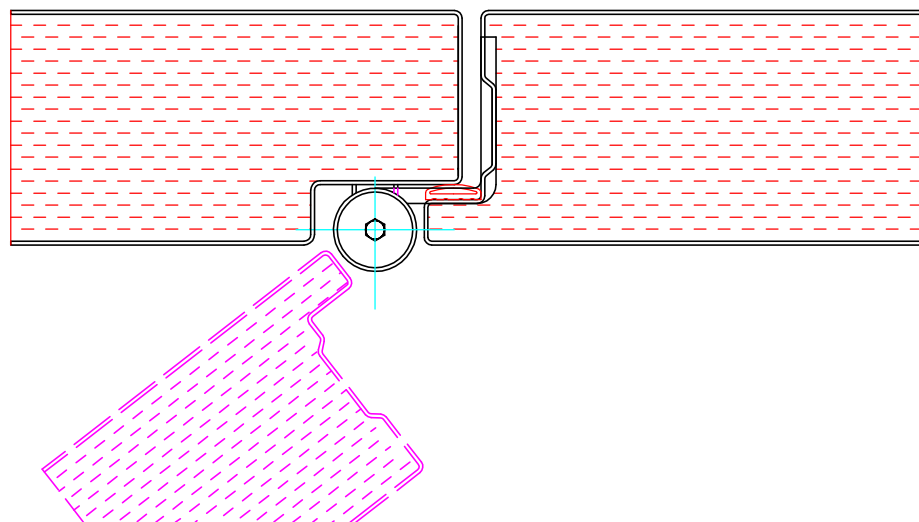
Detail Gehtürband
