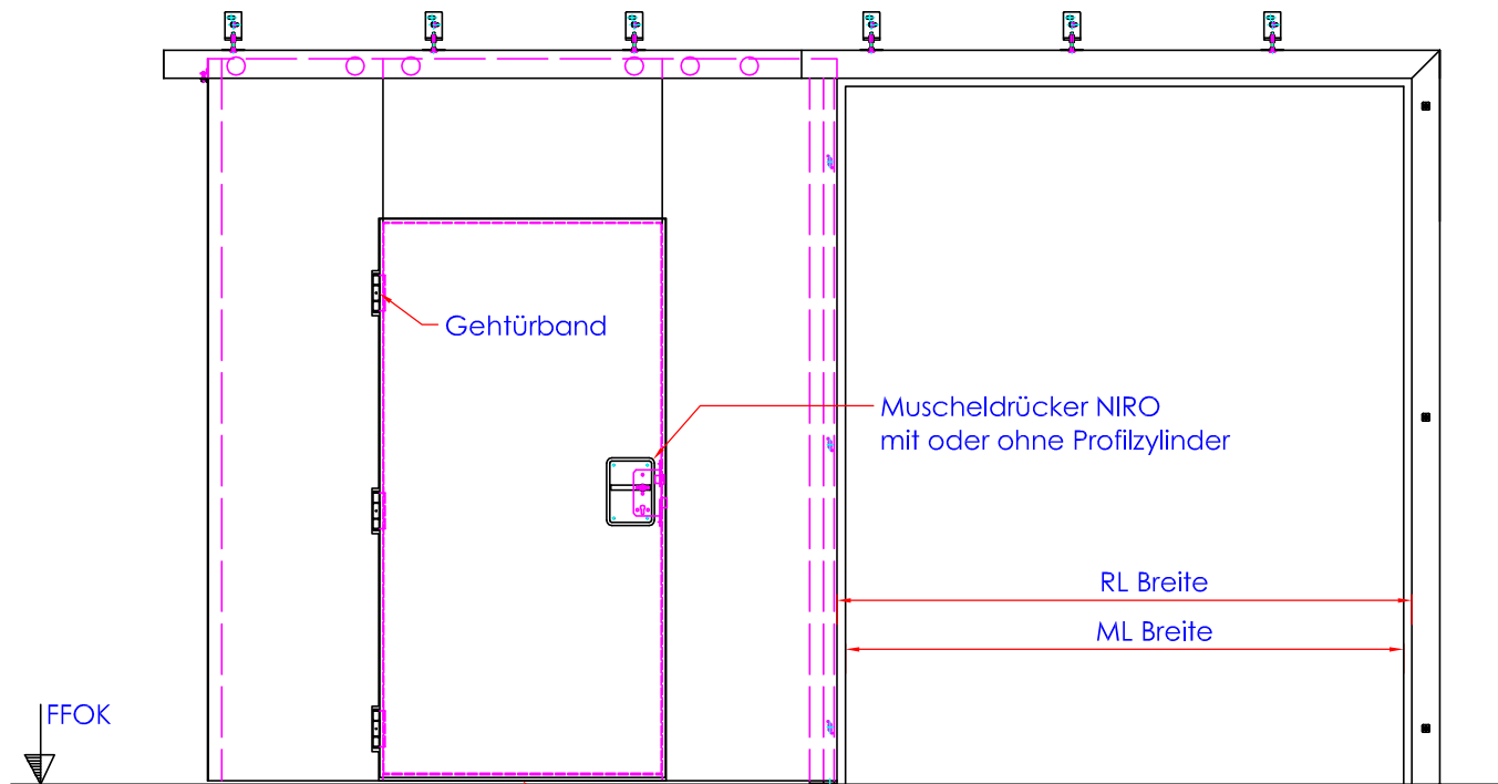
Detail Gehtürband
