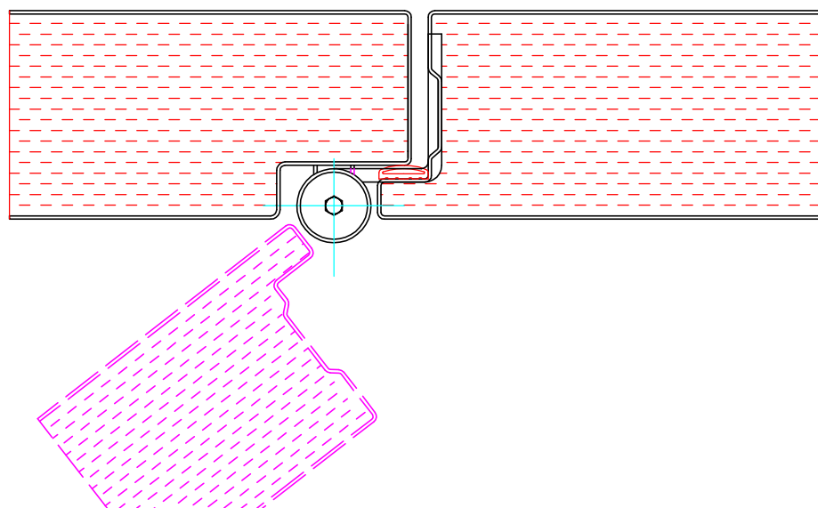
Detail Gehürband
