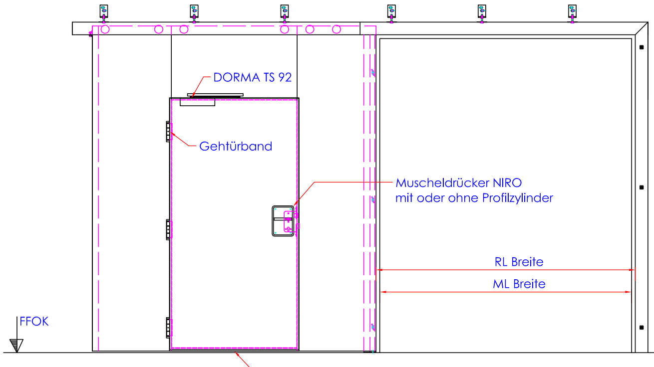
Detail Gehürband
