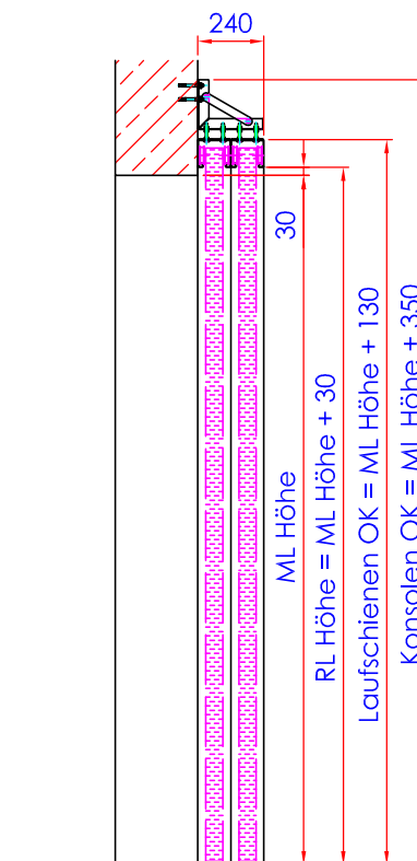
Schnitt A-A
