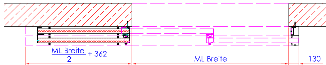
Schnitt B-B
