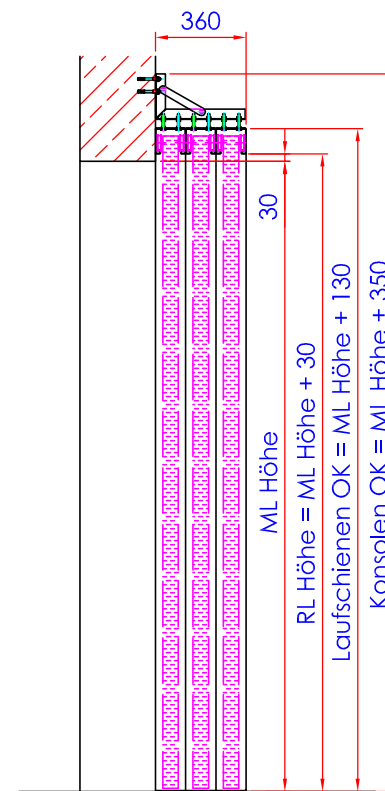
Schnitt A-A
