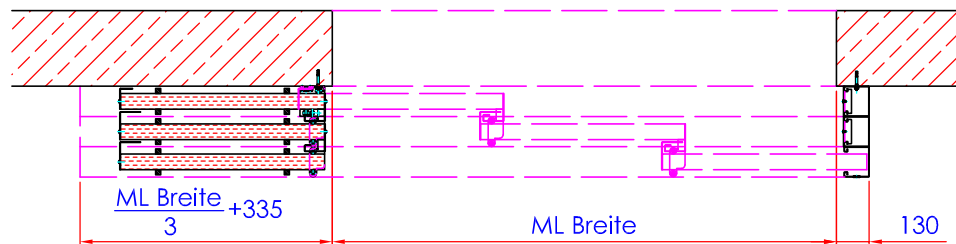
Schnitt B-B
