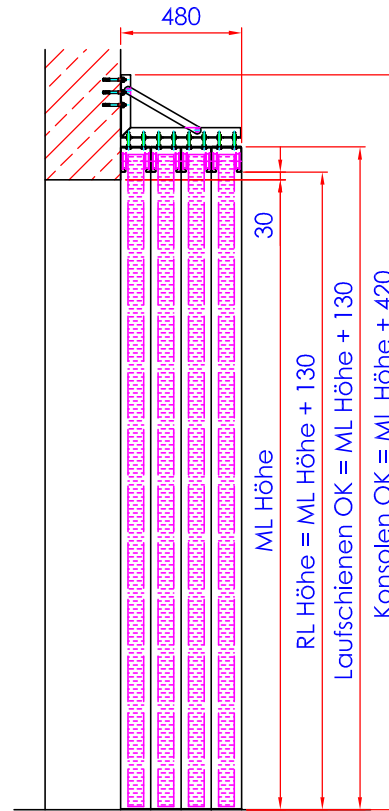
Schnitt A-A
