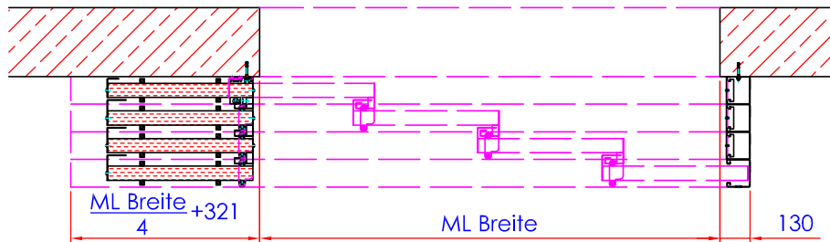
Schnitt B-B
