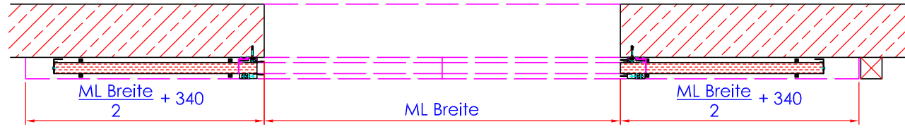
Schnitt B-B
