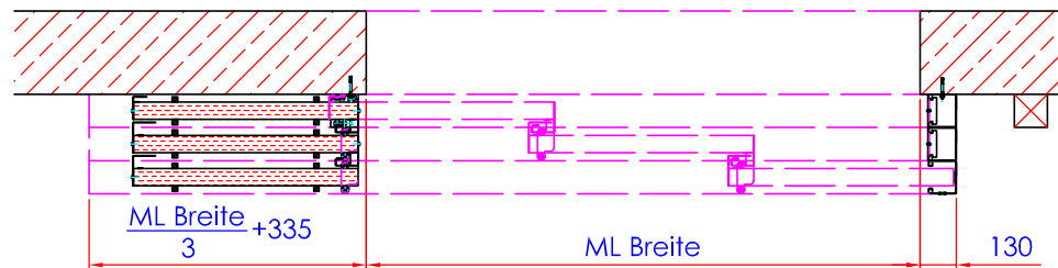
Schnitt B-B
