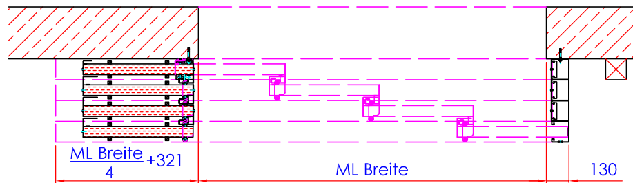
Schnitt B-B
