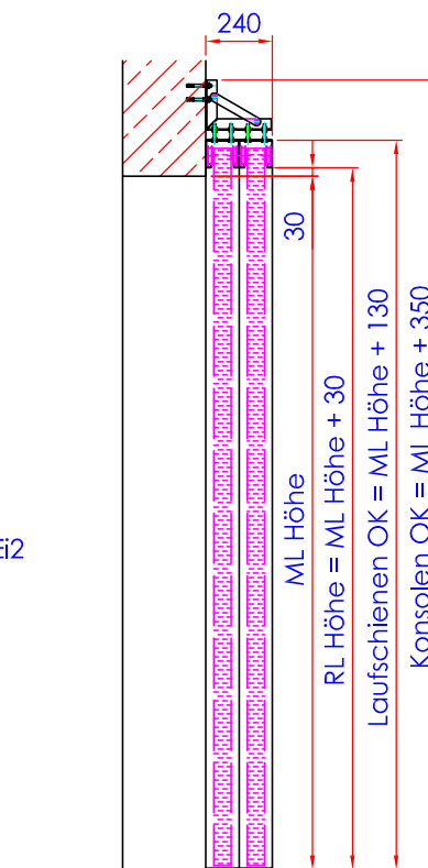
Schnitt A-A
