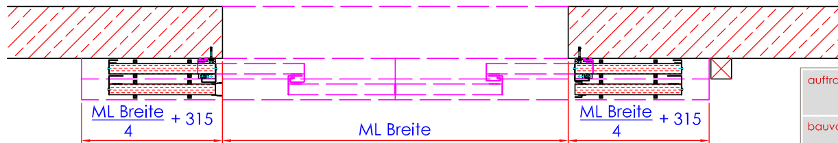
Schnitt B-B
