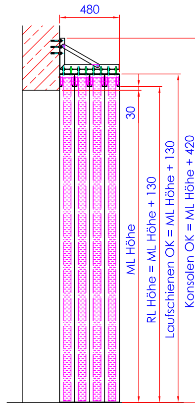
Schnitt A-A
