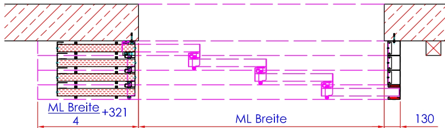
Schnitt B-B
